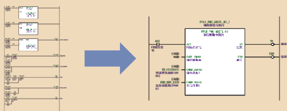
用Function Block重新使用梯形图程序回路
