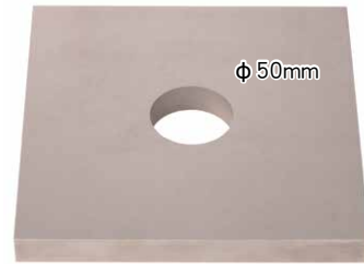
SKD11材20mm厚 \Phi 0.25 黄铜丝 6次加工 \Phi 50mm 真圆度 0.90\mu\text{m}
