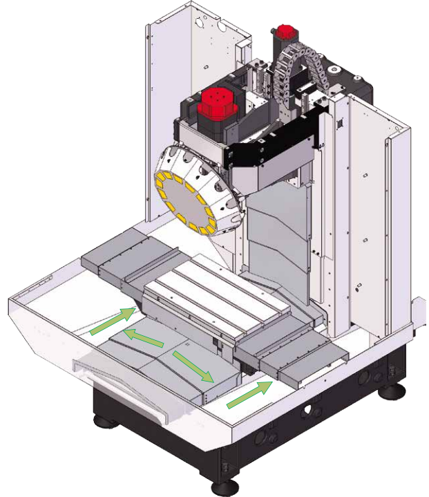
全轴采用可伸缩盖板
