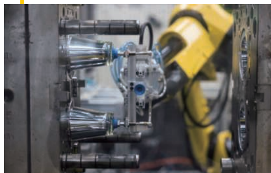
ロボショットでの樹脂成形
