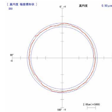
SKD11材20mm厚 φ0.25 黄銅線 6回加工 φ50mm 真円度 0.90μm
