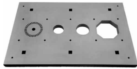
SKD11材30mm厚 φ0.20 黄銅線 5回加工 20mm角穴 ピッチ精度 ±1.1μm
