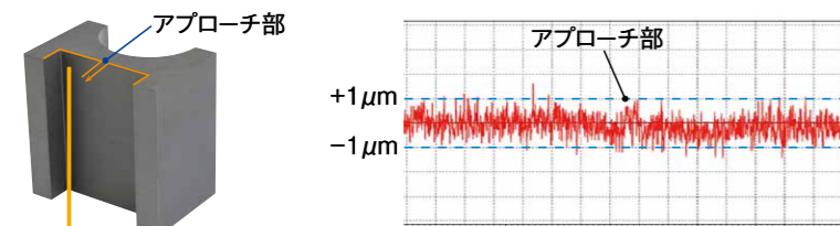
SKD11材30mm厚, φ0.25 黄銅線, 5回加工 形状誤差 ±1μm
