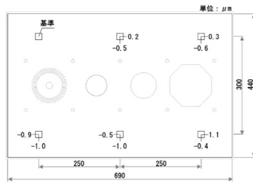
SKD11材30mm厚 φ0.20 黄銅線 5回加工 20mm角穴 ピッチ精度 ±1.1μm
