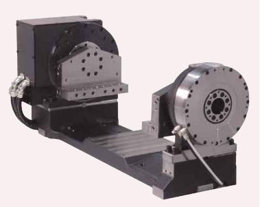
DDR-Ti / DDR-THPi ロボドリルの加工領域を最大限に活かした加工治具を容易に製作可能なユリカゴユニット。クランプトルク1100N・m
