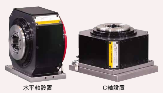
DDR-HSi 高速・高精度位置決めに加え、旋削加工も可能な高速回転タイプ。用途に合わせて設置方向が選択可能です。最高回転数1,500min -1
