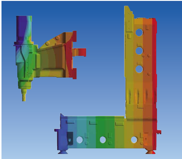
素直に伸びて補正しやすい機構部
