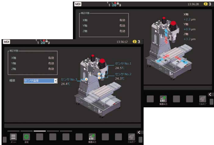
熱変位補正機能画面
