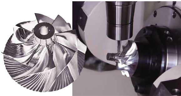
DDモータ仕様2軸テーブルを使用した インペラの高速加工
