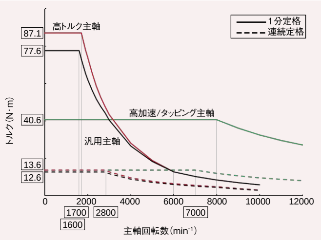
汎用主軸/高トルク主軸/高加速主軸/タッピング主軸
