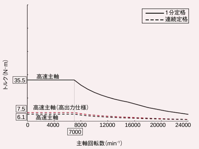
高速主軸
