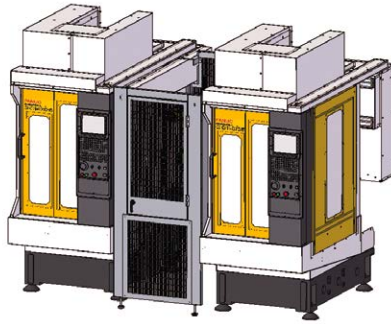
側面一体式 (ロボドリル2台構成)
